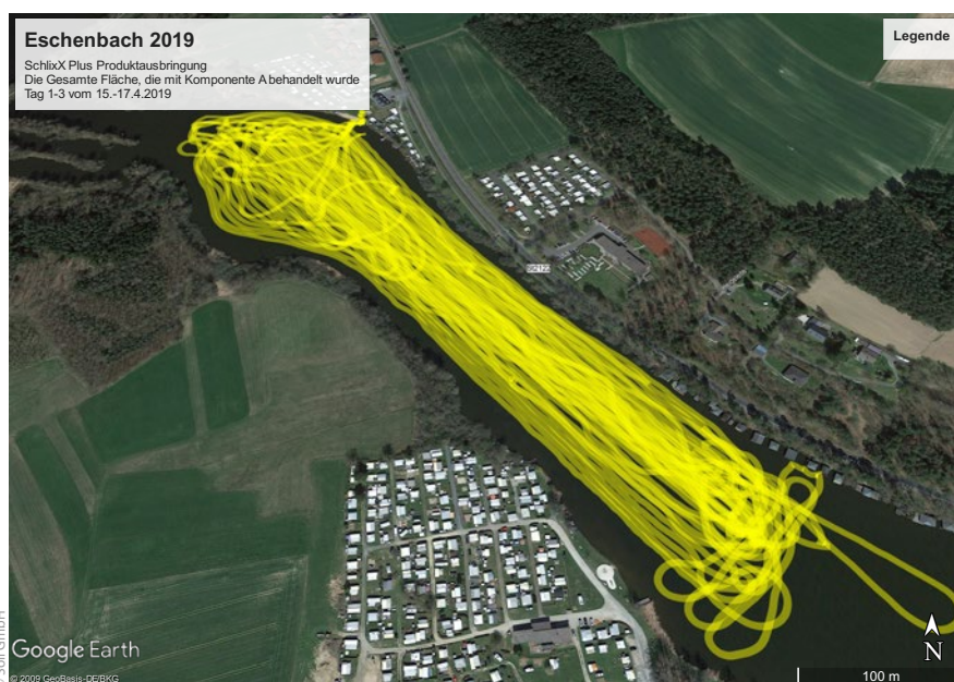
Bild 2: Luftaufnahme des westlichen Teils des Kleinen Rußweiher, die gelbe Linie zeigt die mit GPS erfasste Bootspur der SIP-Applikation über der Sedimentoberfläche
